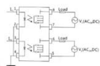
Wiring Diagram 接线图
