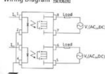
Wiring Diagram 接线图
