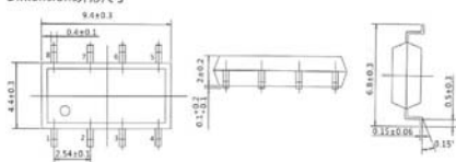
Dimensions 外形尺寸
