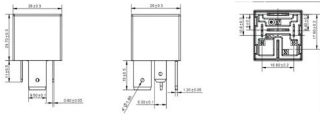
外形图 Outline dimensions
